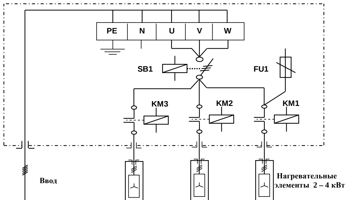
Рис. 8. Силовая схема электродкотла «Daline PTE 10 – 18»
