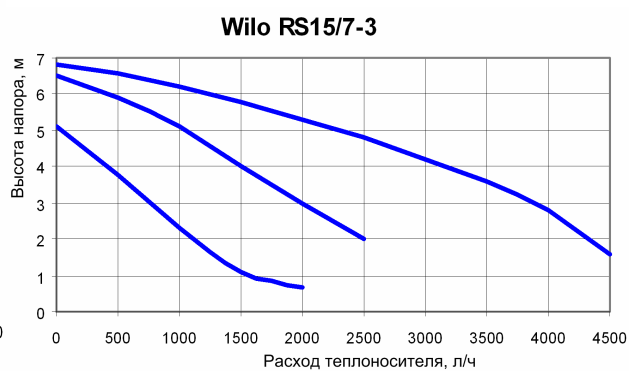
Рис.19. Высота напора насоса «Wilo RS15/7-3»
