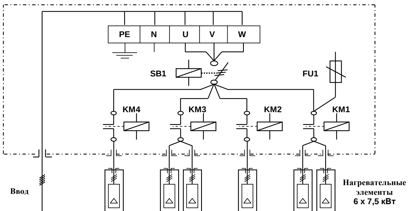
Рис. 11. Силовая схема электродкотла «Daline PTE 45»
