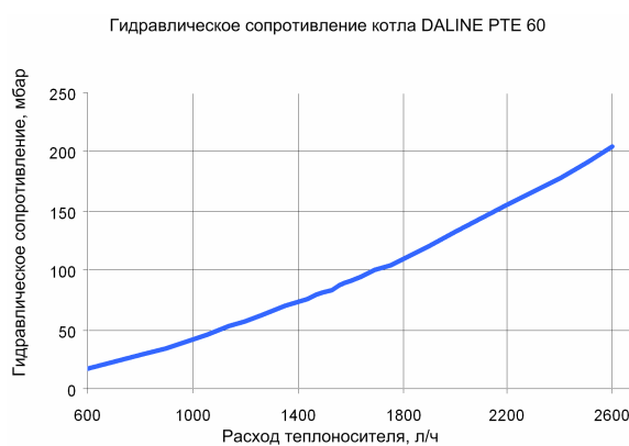
Рис.17. Гидравл. потери котла «Daline PTE 22-60»
