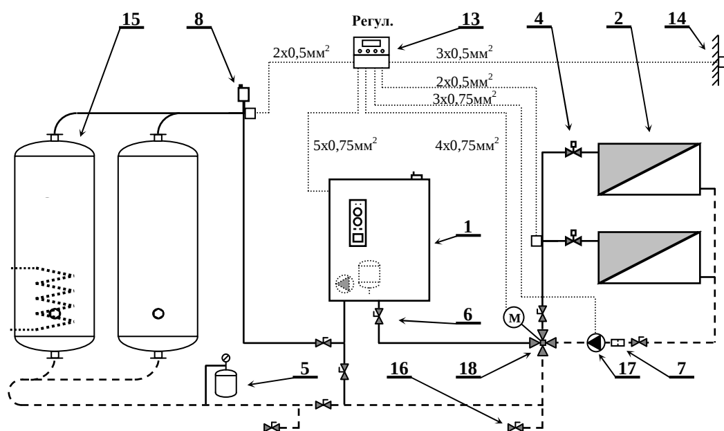
Рис.29. Пример подключения электрокотла к отопительной системе
