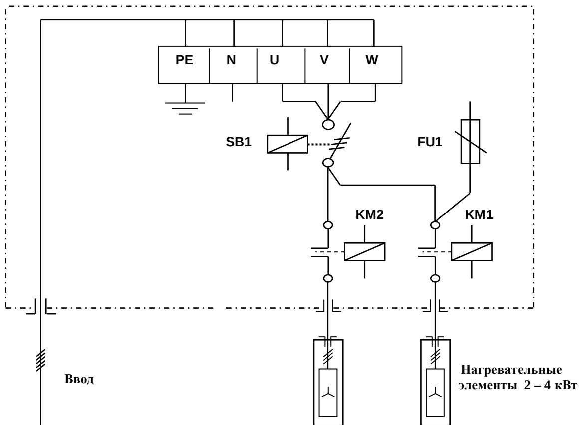
Рис. 7. Силовая схема электродкотла «Daline PTE 4-8»
